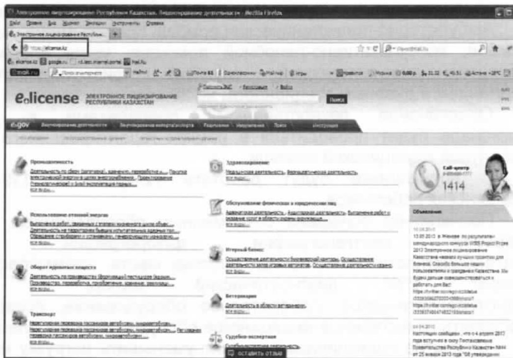
Рисунок 3. Главная страница
